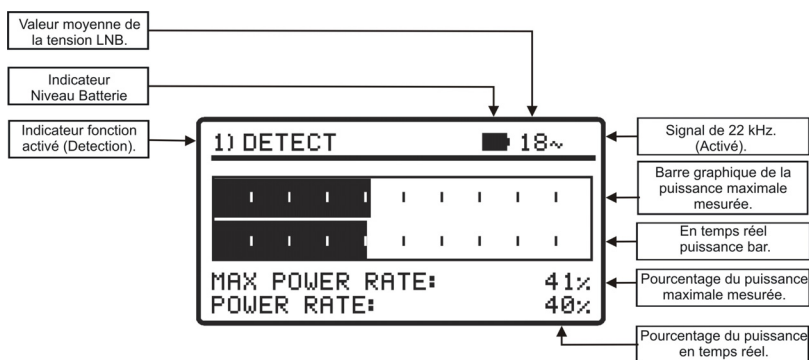
Figure 8.- Écran de la fonction DETECT.
