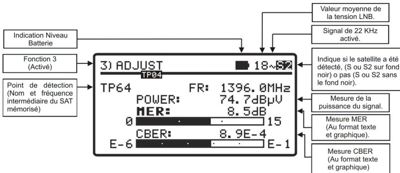
Figure 11.- Écran de la fonction de mesure
