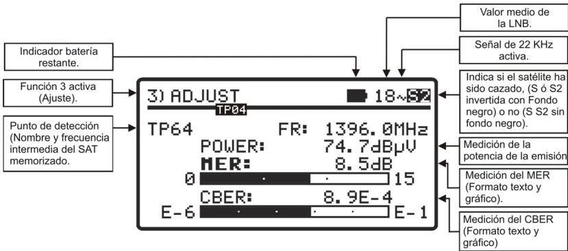
Figura 11.- Pantalla del modo de ajuste.
