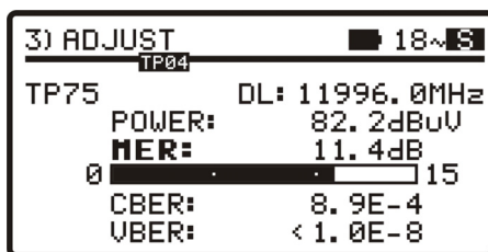
Figure 12.- Écran de mesures de DVB-S avec VBER.
