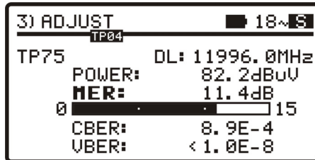
Figura 12.- Pantalla de medidas de DVB-S con VBER.
