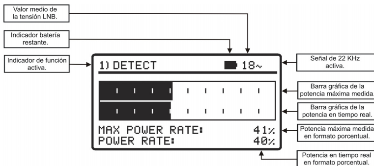
Figura 8.- Función DETECT.
