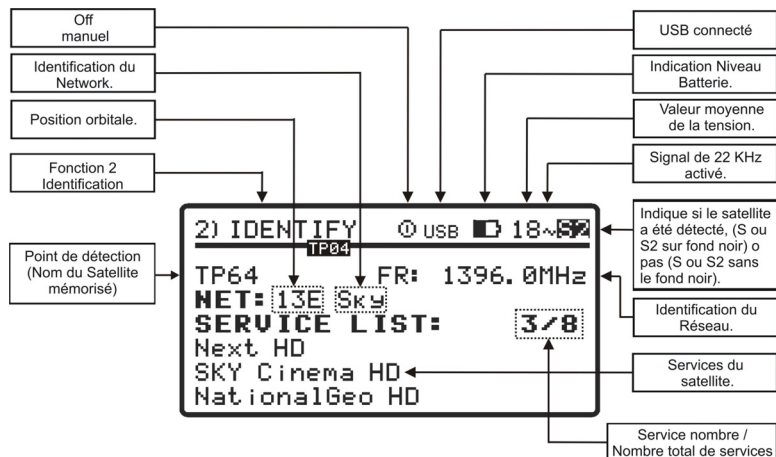
Figure 10.- Écran initiale de la Fonction Identification.
