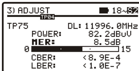
Figura 13.- Pantalla de medida de DVB-S2 con LBER.
