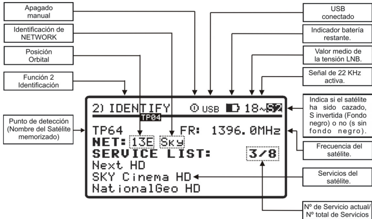
Figura 10.- Pantalla de identificación de un satélite.
