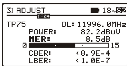
Figure 13.- Écran de mesures de DVB-S2 avec LBER.
